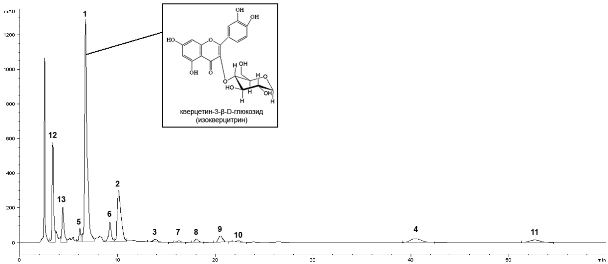
Рисунок 1 – Хроматограмма спиртового извлечения из побегов вереска обыкновенного: 1 – изокверцитрин; 2 – гиперозид; 3 – кемпферол-3-β-D-галактозид; 4 – кверцетин; 5 – рутин; 6 – лютеолин-7-глюкозид; 7,8,10 – не идентифицированный флавоноид; 9 – гербацетин-8-глюкозид; 11 – лютеолин; 12 – хлорогеновая кислота; 13 – 4-гидроксибензойная кислота.
