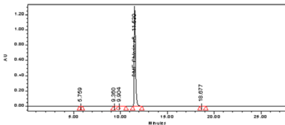
Рисунок 1 – Хроматограмма образца ДМЭ Хеб
