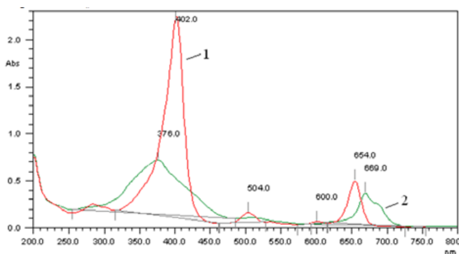
Рисунок 2 – Спектры поглощения хлорина еб (1) и ДМЭ Хеб (2) в буферном растворе Трис 7,4
