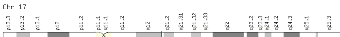
Рис. 3. Локализация гена ErbB- 2/HER2-Neu 17q11.2-q12
