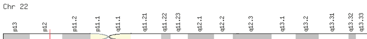
Рис. 5. Локализация гена 18S рРНК
