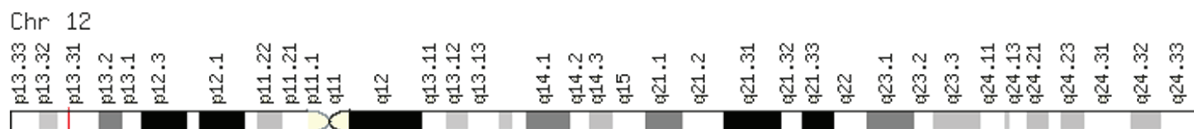
Рис. 4. Локализация гена GAPDH 12p13.31
